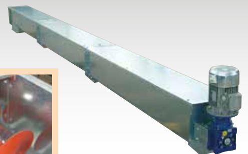
■ Geschlossene Schneckenförderer.
